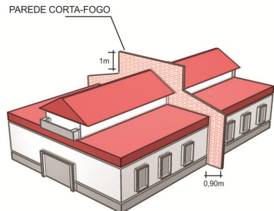
Figura 8 - Parede corta-fogo
